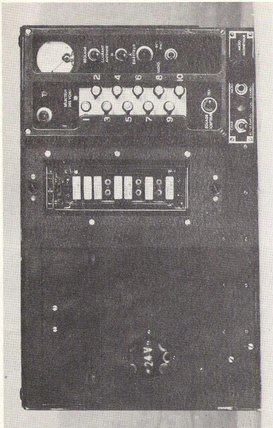
Fig. 3 — Le SCR-508: Emetteur BC-604 (avec version française du répertoriage) La plaque recouvrant les quartz a été enlevée
