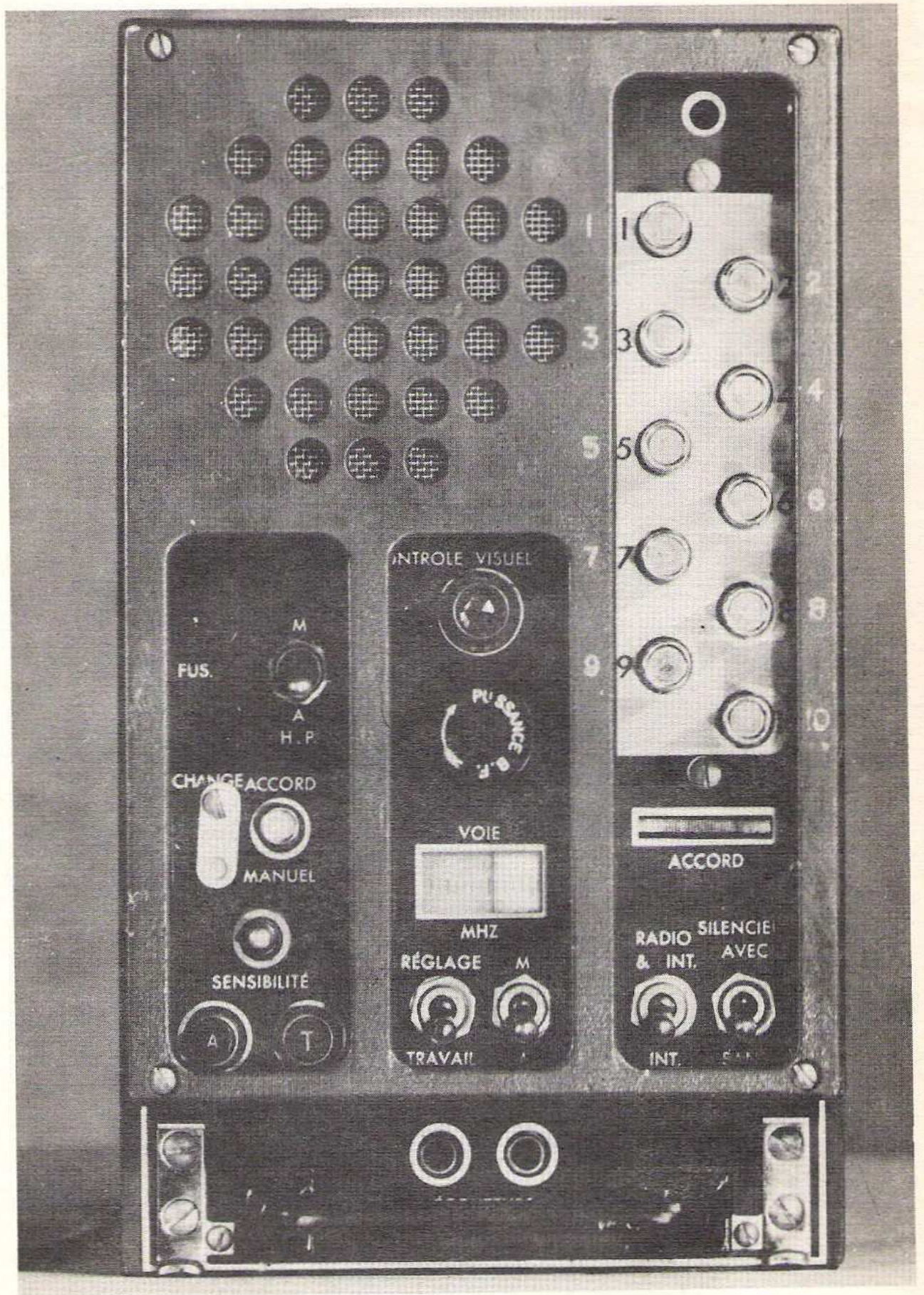
Fig. 4 — Le SCR-508 : Récepteur BC-603 (avec version française du répertoire)
